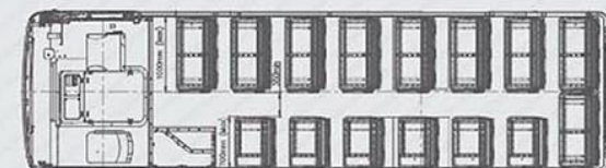
Model : 2075 H Wheelbase : 4320 Seating : 34+D 2X2 41+D 3X2
