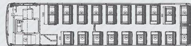
Model : 2090 L Wheelbase : 5240 HHR Seating : 42+D 2X2 51+D 3X2
