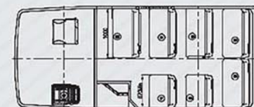
Model : 2050 C Wheelbase : 2850 Seating : 18+D 2X2 21+D 3X2
